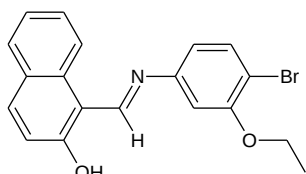
Fig. 2 Secondary ligand 1-{(E)-[(4-bromo-3-ethoxyphenyl)imino]methyl}naphthalen-2-ol
